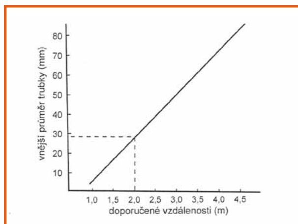
Obrázek 2.4.12 - doporučené vzdálenosti uchycení (podepření) potrubí
