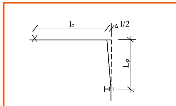
Obrázek 2.4.5 - Předpětí pružného ramena - s předpětím \Delta l/2
