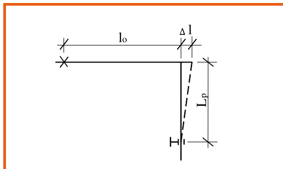
Obrázek 2.4.4 - Předpětí pružného ramena - bez předpětí
