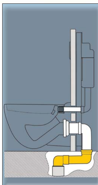
Art. OHA.3983 WC prodloužení ploché DN 110 nastavitelná délka 15-35 cm výška zapuštění v podlaze pouze 85 mm !!!
