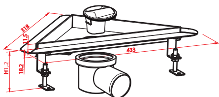
art. PB.SYK0300 rohový odtok do prostoru
