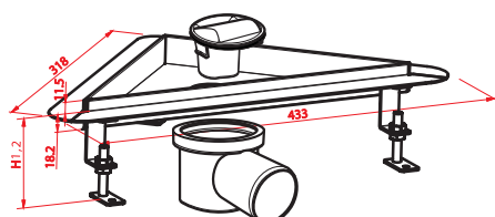
art. PB.SYK0300 rohový odtok do prostoru
