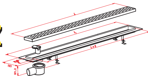
art. PB.SZK0600 (0700, 0800, 0900, 1000) odtokový žlab do prostoru
