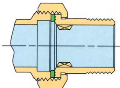
Art. CLF.588xxx 3 dílné šroubení pro solární systémy T max = 160°C, P max = 16 bar maximální obsah glycolu v médiu 50%
